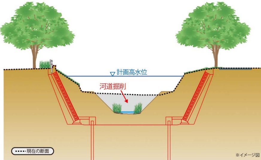
5 6 図 2-7 河道断面イメージ
