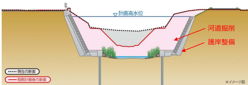
12 13 図 2-8 河道断面イメージ
