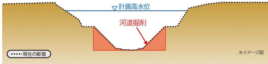
8 図 2-3 河道掘削イメージ
