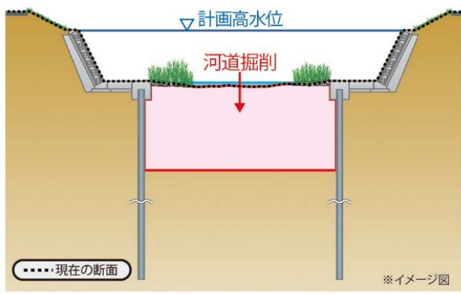
5 6 図 2-9 河川改修イメージ 7
