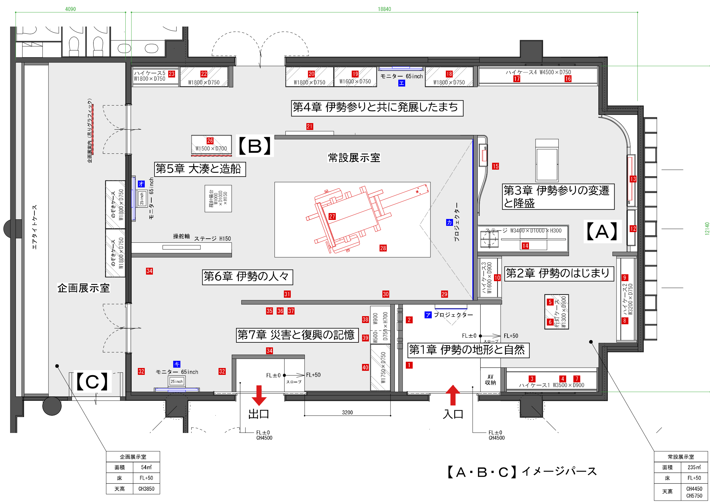
伊勢市歴史博物館 常設展示室・企画展示室 詳細平面図
