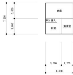
業務員室棟 平面図 1:300
