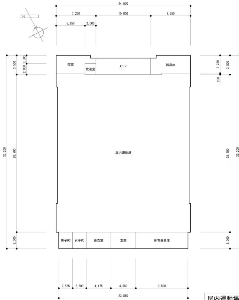
屋内運動場棟 平面図 1:300
