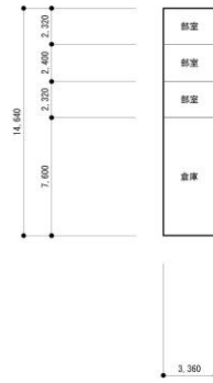
部室・倉庫棟 平面図 1:300
