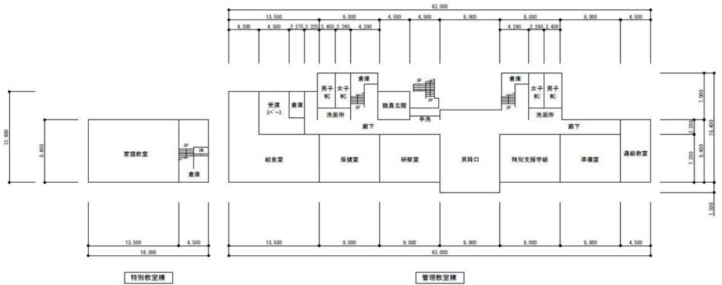
校舎 1階平面図
