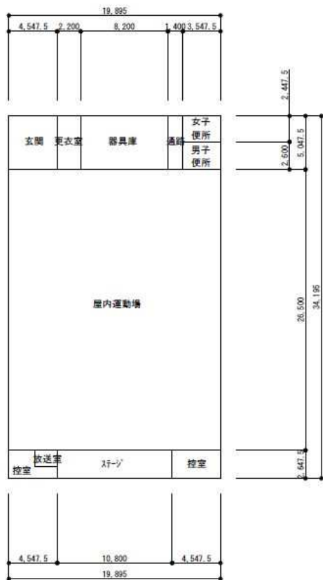
屋内運動場 1階平面図
