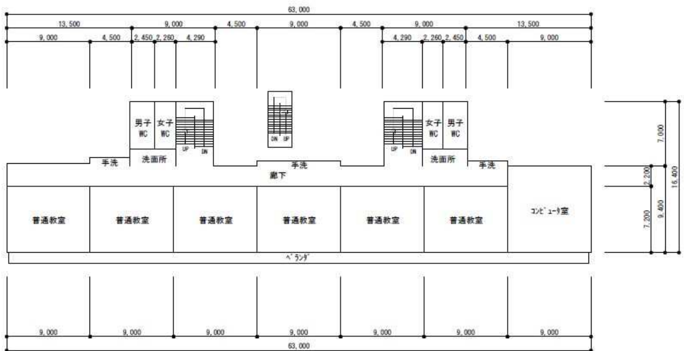
校舎 3階平面図
