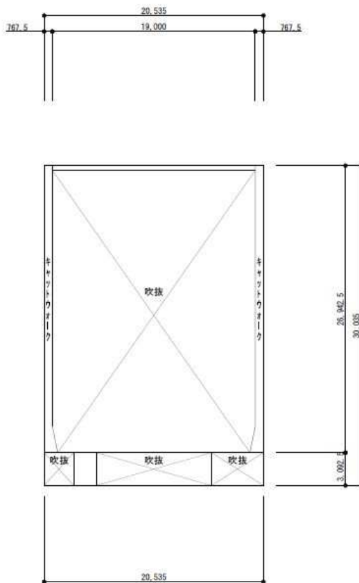
屋内運動場 上部平面図
