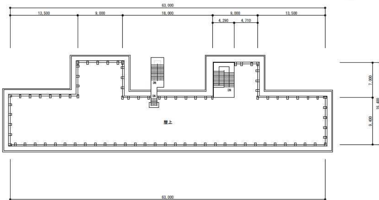
校舎 屋上平面図
