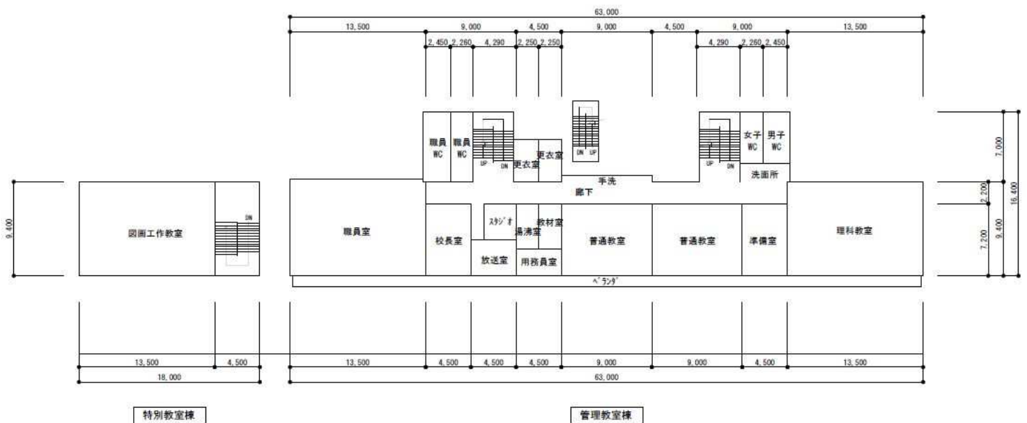
校舎 2階平面図
