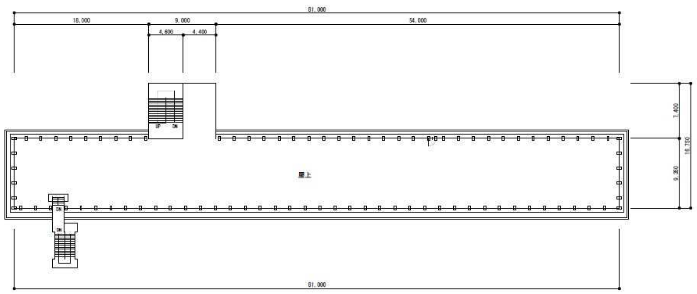
校舎 屋上平面図
