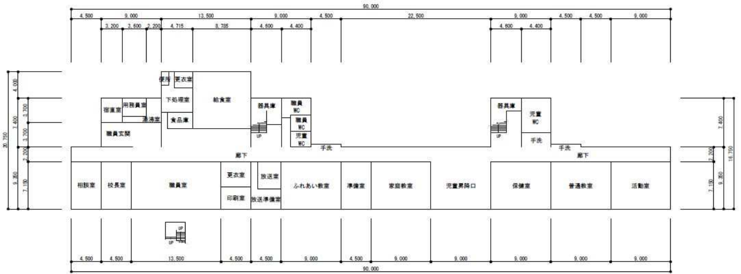
校舎 1階平面図
