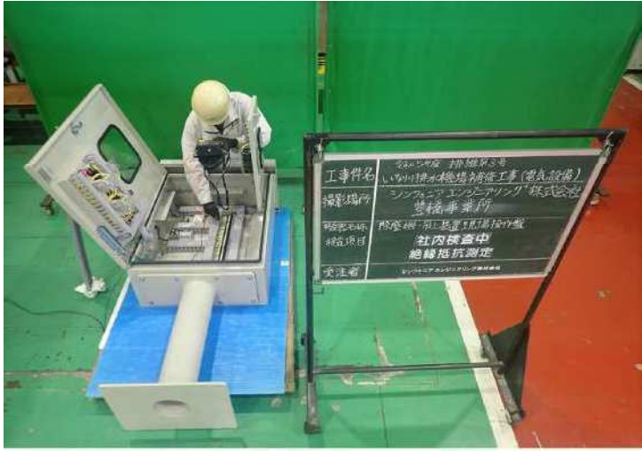
施工状況
