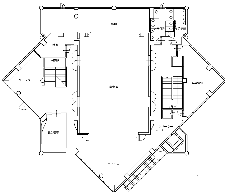
2階 平面図 1/300
