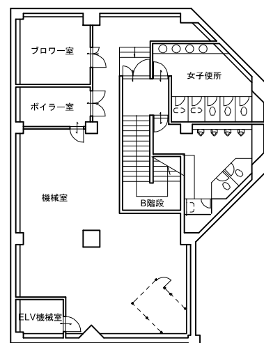
地階 平面図 1/300
