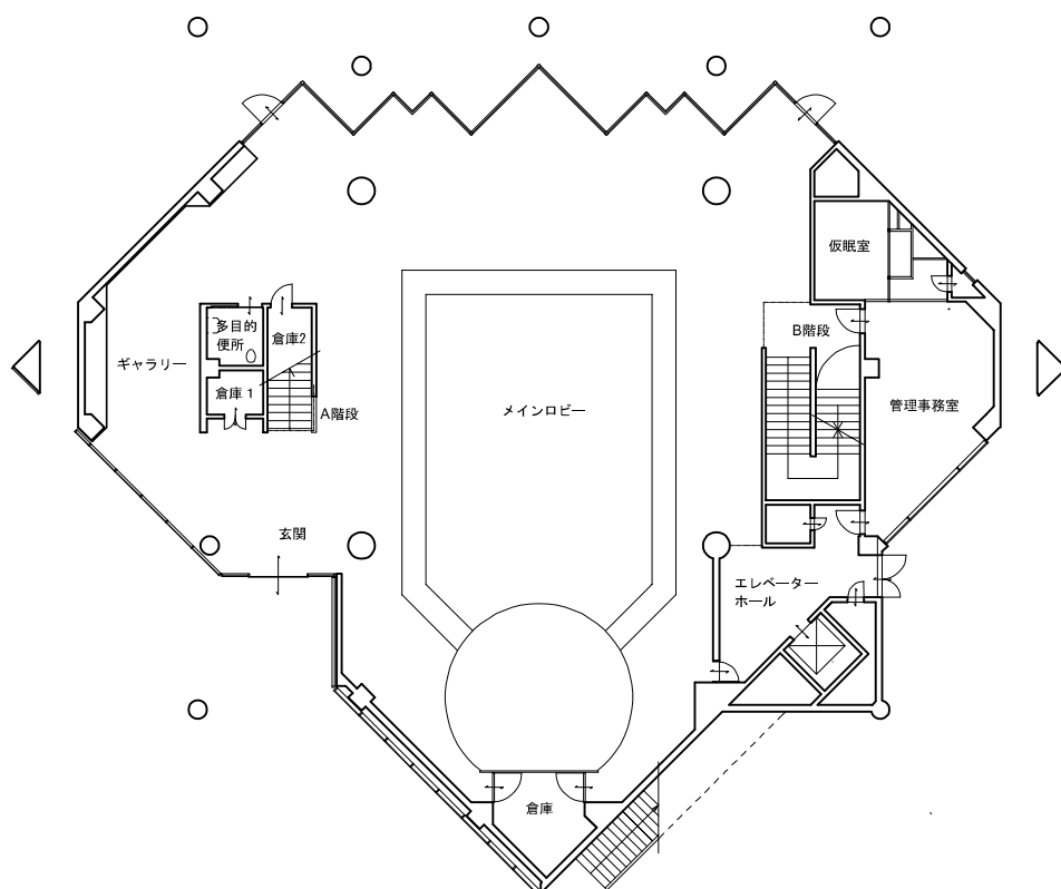
1階 平面図 1/300
