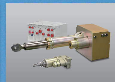
宇宙ロケット姿勢制御用サーボアクチュエータ
