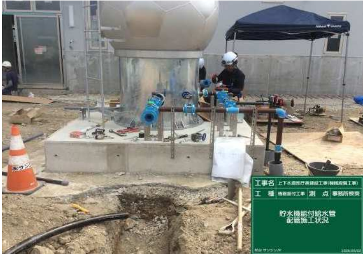
施工状況
