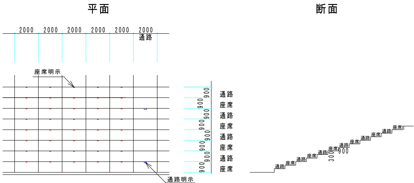
2人席詳細図（階段部） S=1:200
