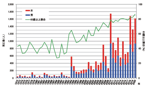
年次別男女別熱中症死亡数(1972~2020年)
