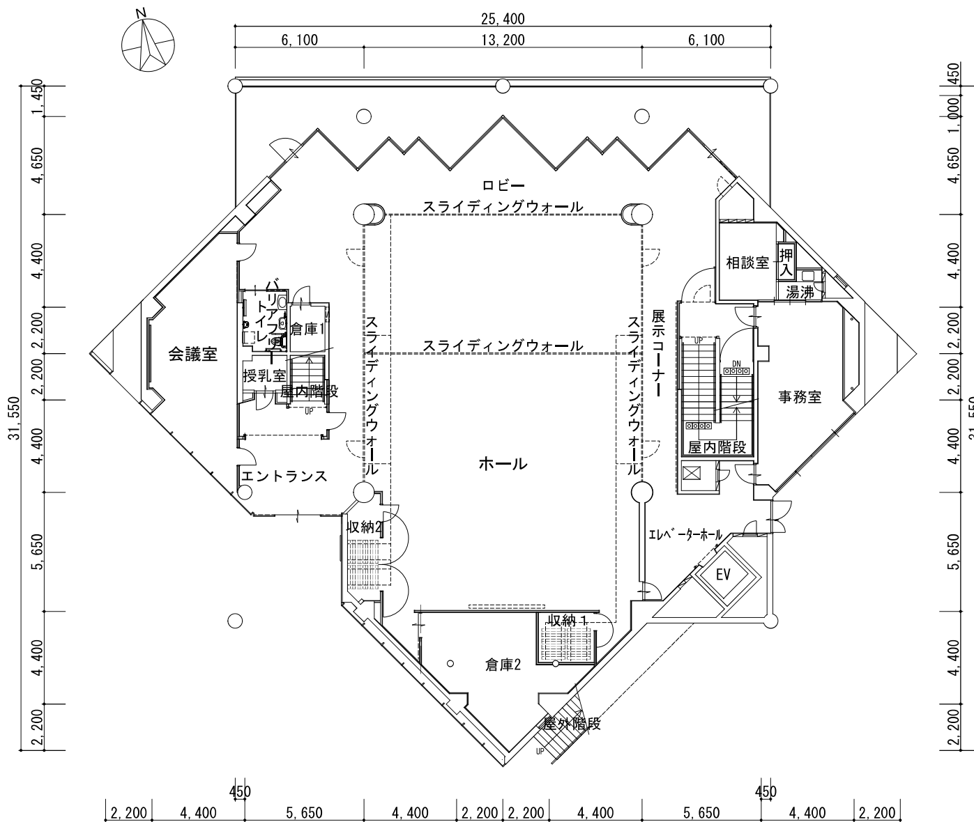
北館1階平面図
