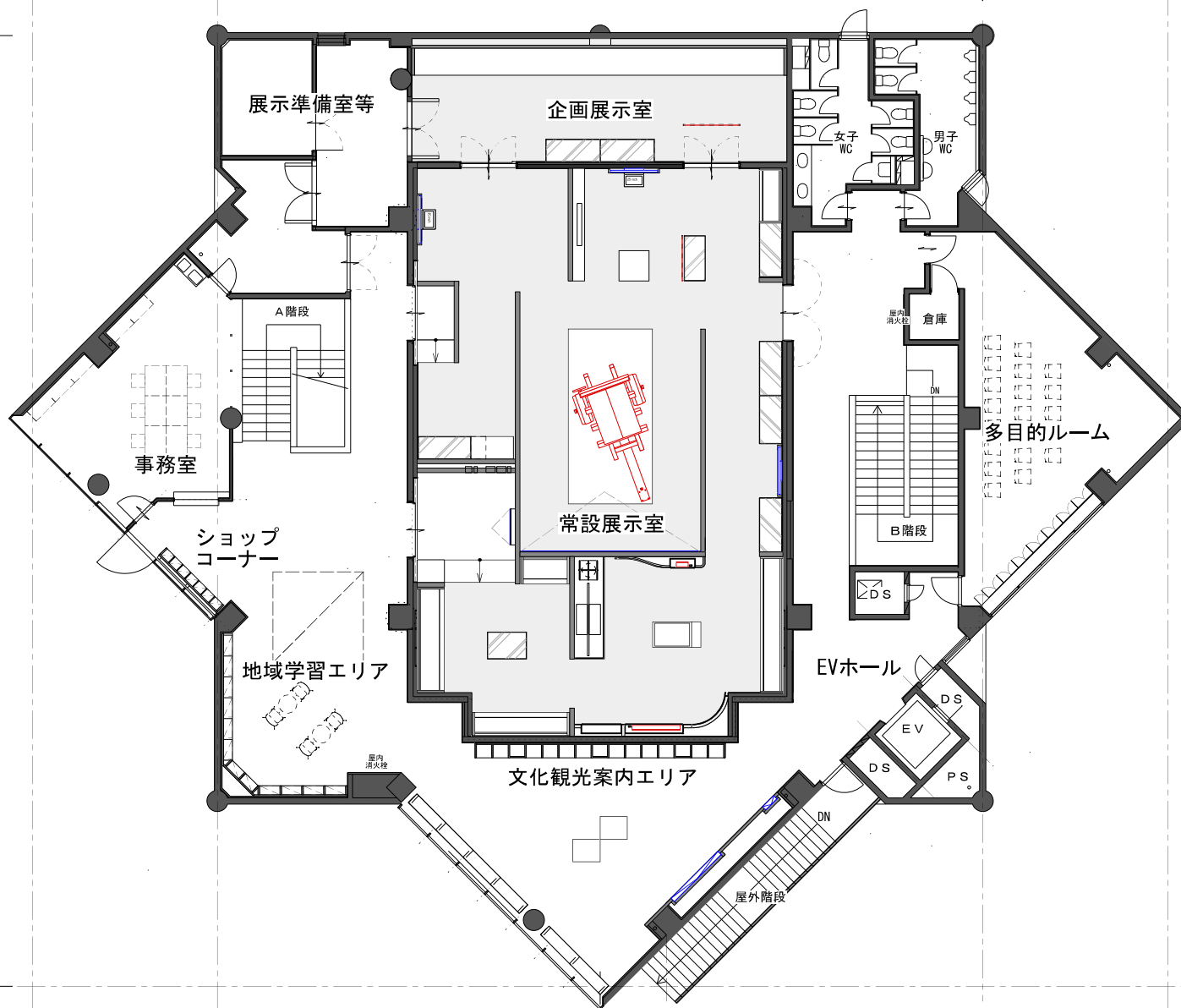
北館2階 全体平面図
